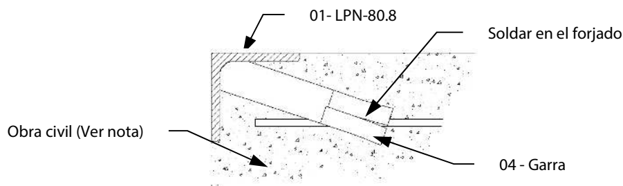
Detalle A del premarco
